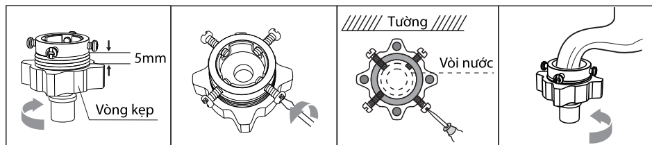
Nới lỏng vòng kẹp để phần ren rộng 5 mm
