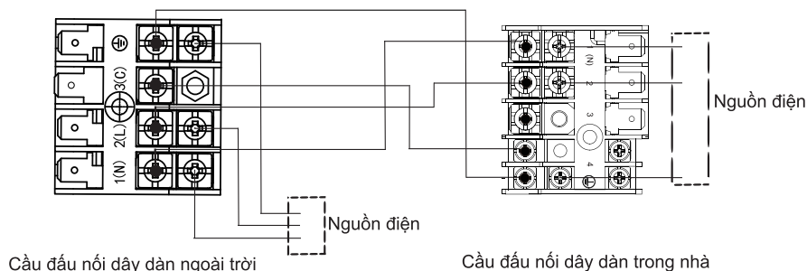
Sơ đồ mạch (Cấp nguồn dàn trong nhà hoặc dàn ngoài trời)
