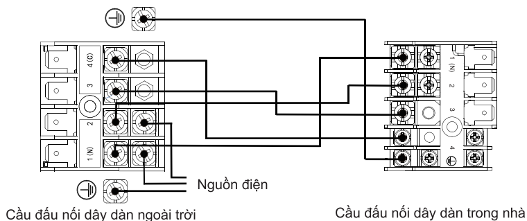
Sơ đồ mạch (Cấp nguồn từ dàn ngoài trời)
