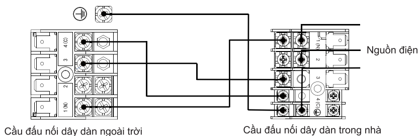
Sơ đồ mạch (Cấp nguồn từ dàn ngoài trời)
