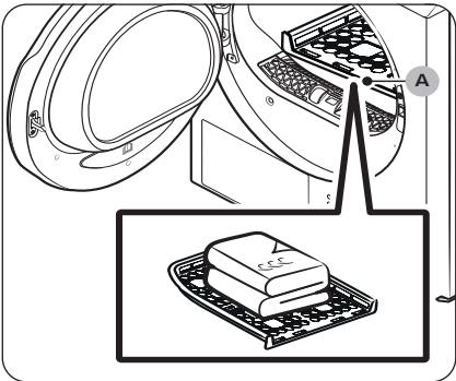
A. Dàn sấy
