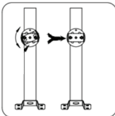
2. Điều chỉnh góc độ: Thanh nối có thể xoay trên đế tròn của giá đỡ. Khi xoay đến góc độ thích hợp theo nhu cầu lắp đặt, cố định bằng vít.
