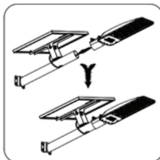
6. Luồn dây đầu ra của tấm pin năng lượng mặt trời qua lỗ ở dưới cùng của giá đỡ, kéo nó ra khỏi mặt trước và kết nối nó với đường dây đầu vào của đèn đường, sau đó cố định giá đỡ bằng vít và thu gọn phần dây còn dư vào khung giá đỡ.
