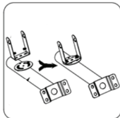
1. Đặt đai ốc và vít vào thanh nối và giá đỡ. Lưu ý: Chỉ lắp vít vào, chưa siết chặt.
