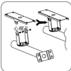
3. Luồn các vít xuyên qua các lỗ vít trung tâm của giá đỡ tẩm pin và thanh nối giá đỡ. Lưu ý: Không cần siết chặt vít ở bước này.
